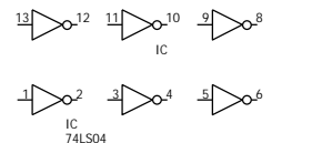
Fig11: TTL INVERTER
