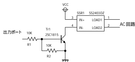
Fig2: SSRによるAC回路ON/OFF
