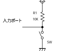
Fig7: スイッチ入力回路
