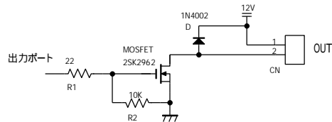
Fig3: DCモーターON/OFF回路
