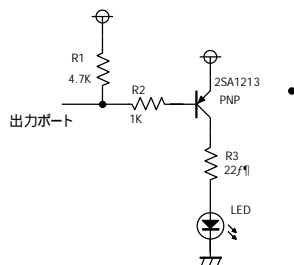
Fig6: 大電流LEDドライブ
