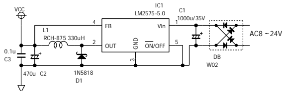
Fig8: 5端子レギュレーター
