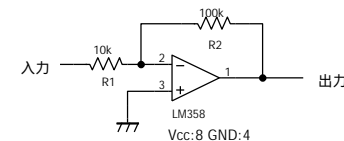
Fig16: OPアンプ反転増幅回路
