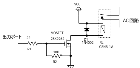
Fig1: リレーによるAC回路ON/OFF
