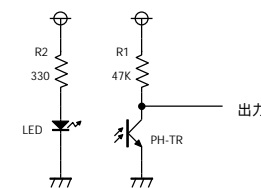
Fig15: フォトトランジスタ回路
