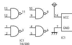
Fig10: TTL NAND
