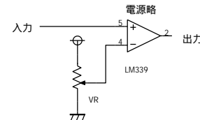
Fig13: コンバーター
