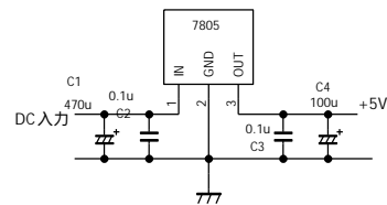
Fig9: 3端子レギュレーター
