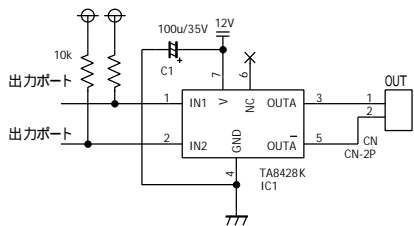
Fig6: 大電流LEDドライブ
